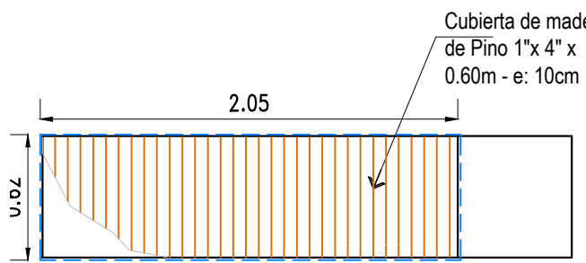
CUBIERTA STAND - ESC 1:100
