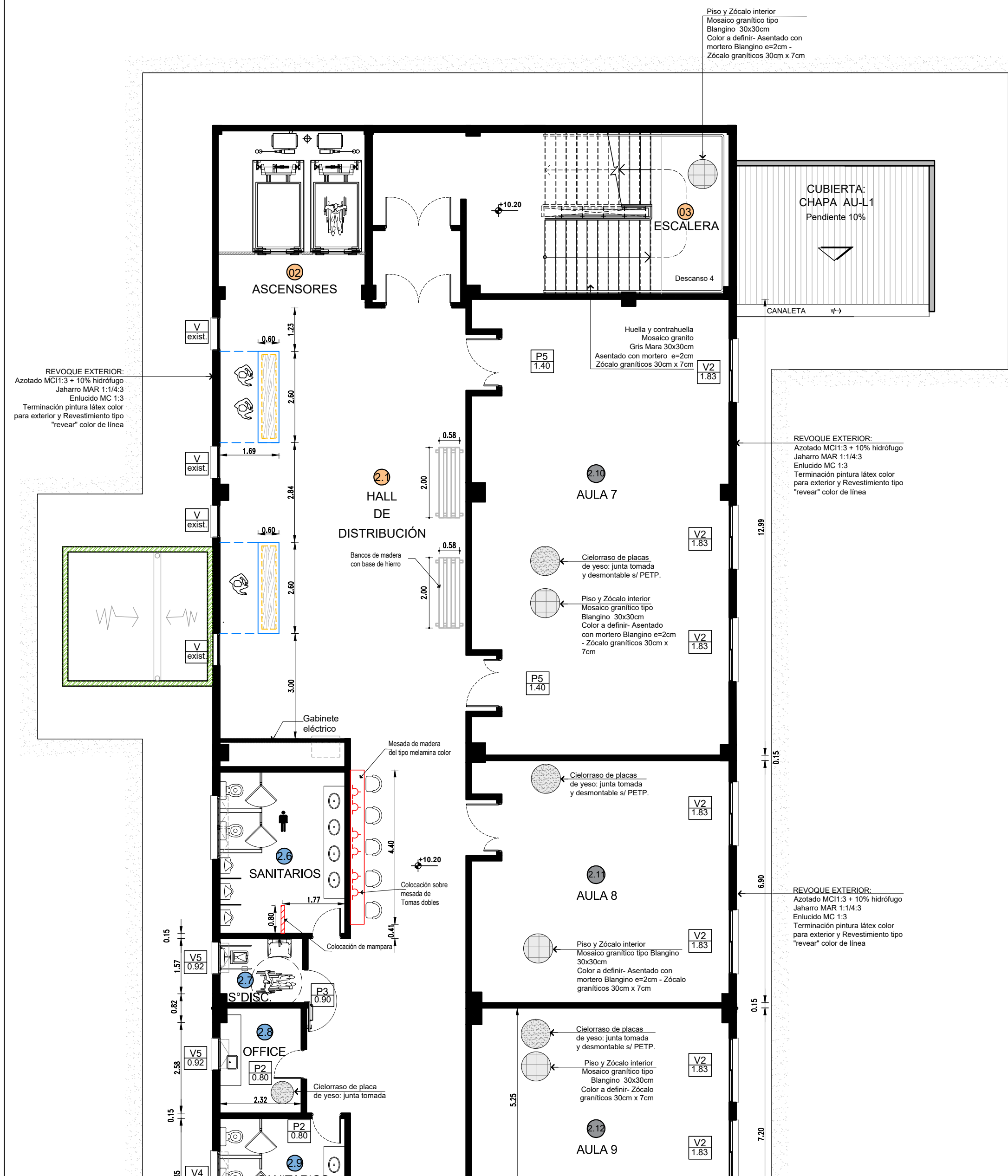
PROPUESTA STAND AGRUPACIONES_ 2º Piso ESC 1:100
