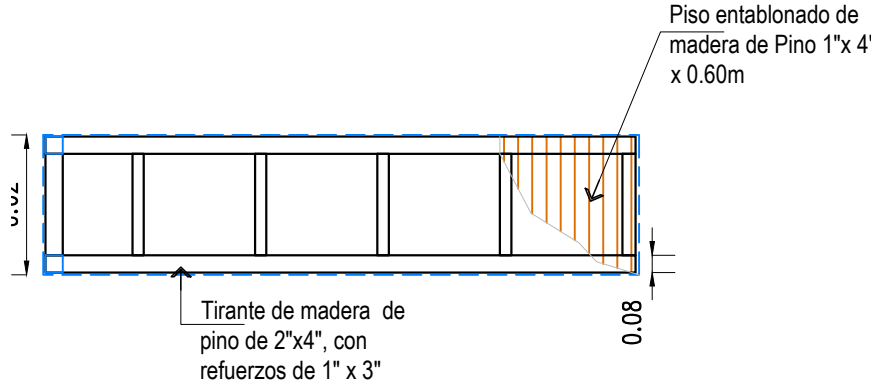
ESTRUCTURA STAND - ESC 1:50
