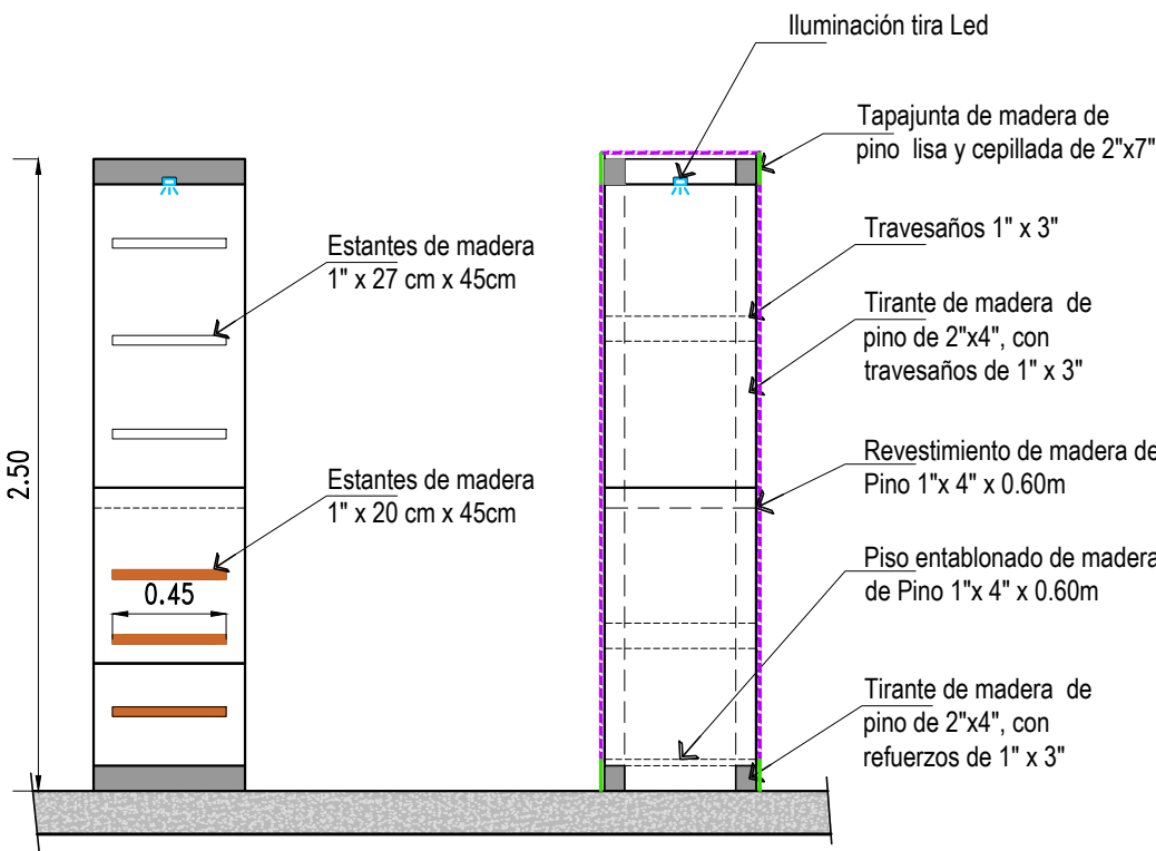
VISTA ESTRUCTURA STAND - ESC 1:50
