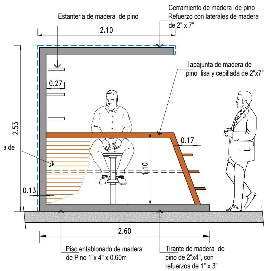
VISTA STAND - ESC 1:50
