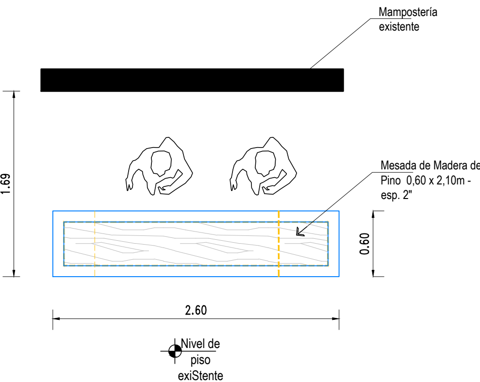
PLANTA STAND AGRUPACIONES - ESC 1:50
